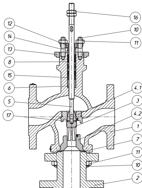
Rys. 1. Zawór regulacyjny
