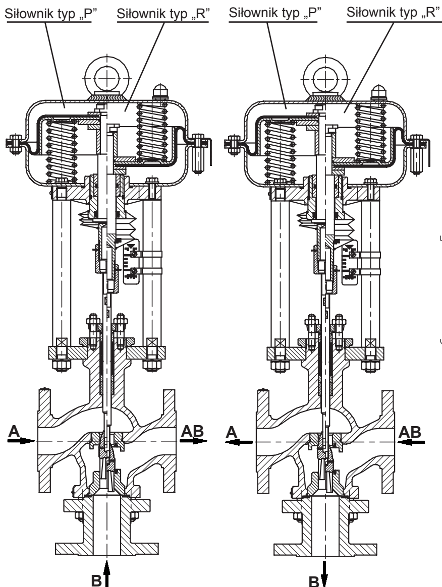
Rys.3. P/R-Z3M - Mieszający
