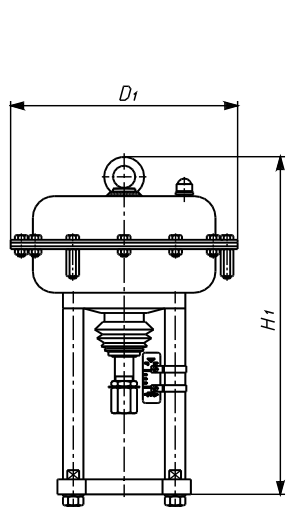
Rysunek 6. Siłowniki typ P/R, PN/RN
