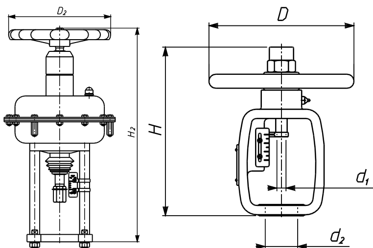
Rysunek 7. Napęd ręczny typ 20.
