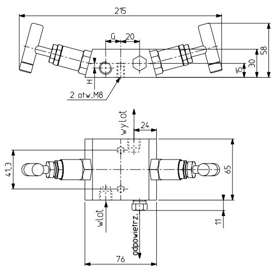
ZA - 24 - zawór iglicowy (jak ZA - 23), z gwintem wewnętrznym na wlocie i wylocie.
