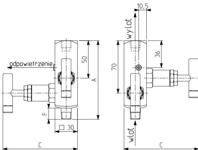
ZA - 22 - zawór iglicowy (jak ZA - 21), z gwintem zewnętrznym na wlocie i wewnętrznym na wylocie.
