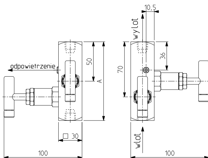
ZA - 21 - zawór iglicowy, podwójny - odcinający i odpowietrzający, liniowy, z gwintami wewnętrznymi na wlocie i wylocie.
