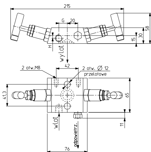
ZA - 23 - zawór iglicowy, podwójny - odcinający, z odpowietrzeniem, blokowy, z gwintem wewnętrznym na wlocie i przyłączem kołnierzowym na wylocie.
